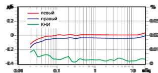
АЧХ/КНИ аналогового аудиотракта
